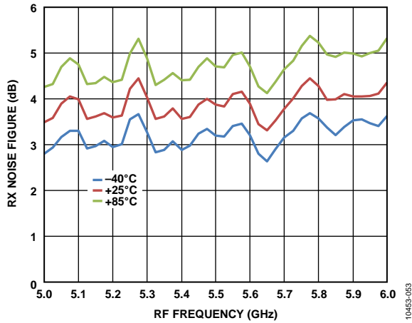
图53. RX噪声系数与RF频率的关系
