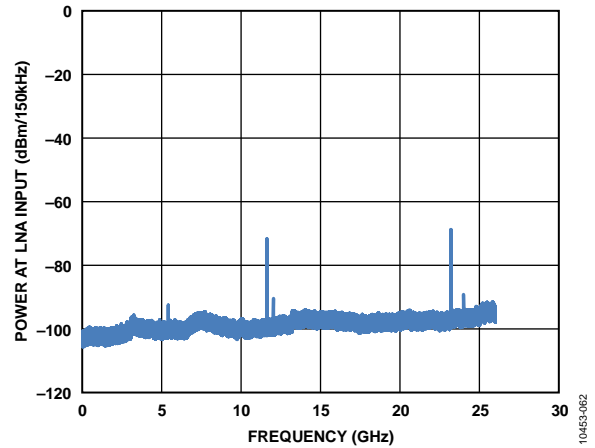
图62.LNA输入端的RX发射(直流至26 GHz, f_{LO\_RX} = 5.8 \text{ GHz} , WiMAX 40 MHz)
