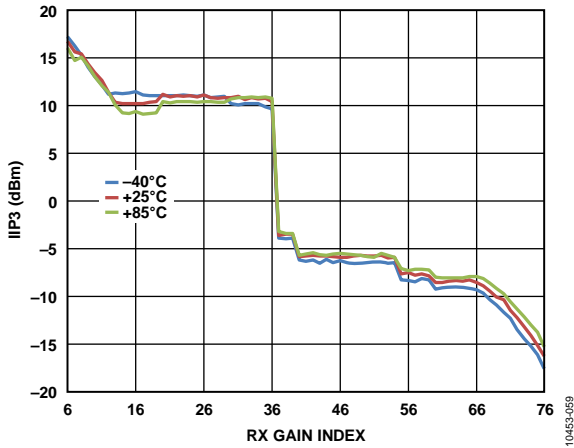
图59.三阶输入交调截点(IIP3)与增益指数的关系 ( f_1 = 50 \text{ MHz} , f_2 = 101 \text{ MHz} )
