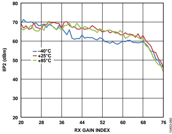
图60.二阶输入交调截点(IIP2)与增益指数的关系 ( f_1 = 70 \text{ MHz} , f_2 = 71 \text{ MHz} )
