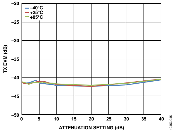
图45. TX EVM与发射器衰减设置的关系 (40 MHz REF_CLK, LTE 20 MHz, 64 QAM调制)
